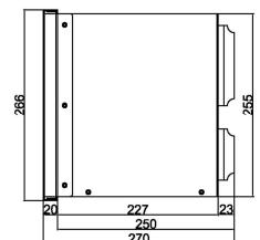
[측면도]
