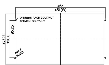
[판별 가공도]
