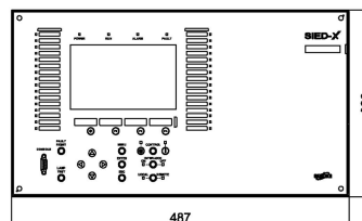
[정면도]
