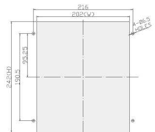
[판넬 가공도]
