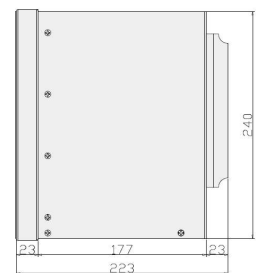
[측면도]
