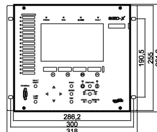
[ 정면도 ]
