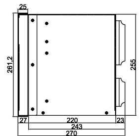
[ 측면도 ]
