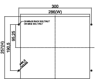
[ 패널 가공도 ]
