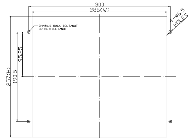
[판넬 가공도]
