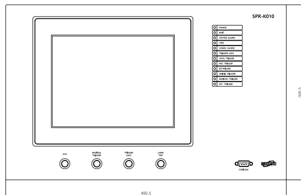
[정면도]
