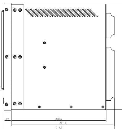
[측면도]
