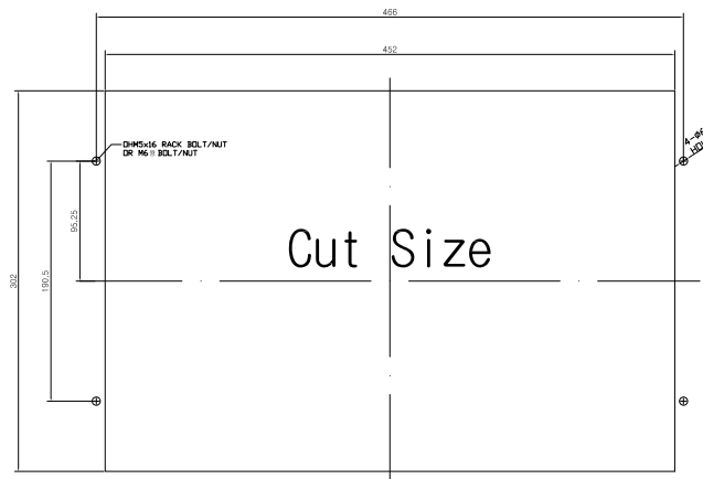
[판넬 가공도]
